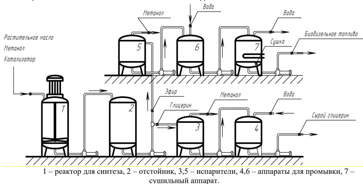
Рисунок 3 – Аппаратурное оформление традиционного процесса получения биодизельного топлива
