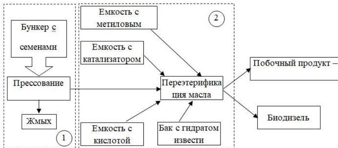
Рисунок 2 – Схема получения метиловых эфиров
