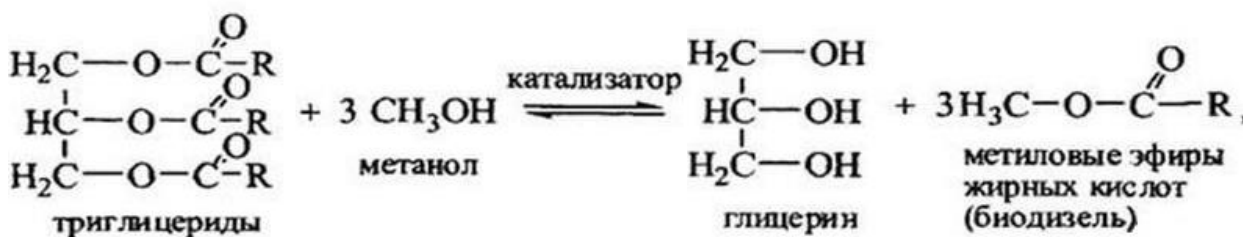
Рисунок 2 – Реакция метанолиза
