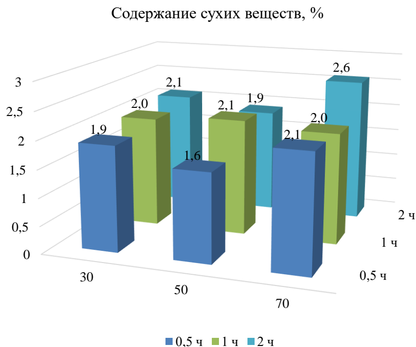
Рисунок 2 – Диаграмма содержания сухих веществ в растительных экстрактах
