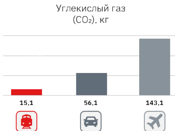
Рисунок 2 – Соотношение выбросов парниковых газов различными видами транспорта (маршрут Москва – Нижний Новгород)
