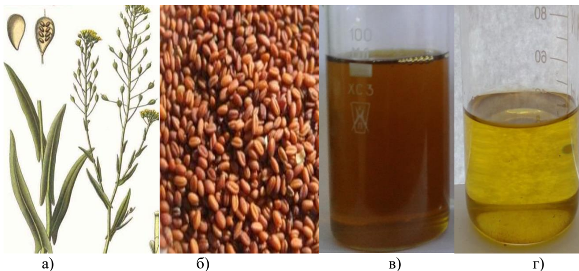
Рисунок 3 – Внешний вид рыжика ярового (а), его семян (б), масла (в) и метиловых эфиров масла (г)
