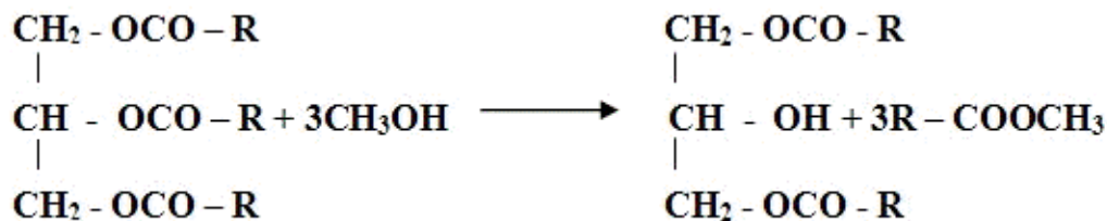
Рисунок 1 – Получение метиловых эфиров по реакции переэтерификации
