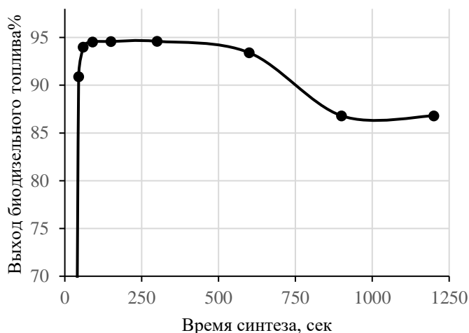
Рисунок 5 – Влияние времени обработки на выход готового продукта
